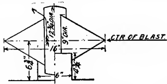
Fig. 4316. THE TORPEDO.
